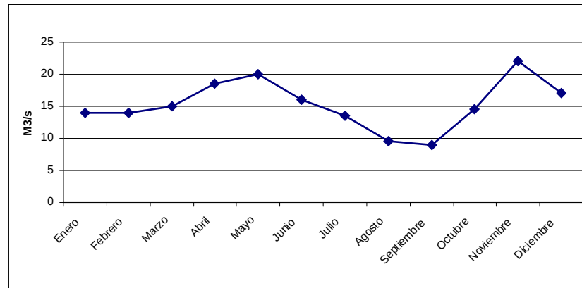
Gráfica 2. Caudal del río Tulúa
