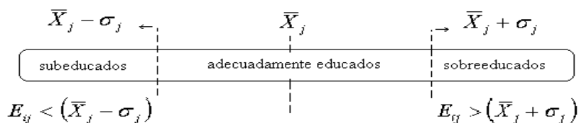
Esquema 5.1: Método estadístico
